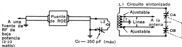
Fig. 6-4. Ajuste del acoplador de antena
