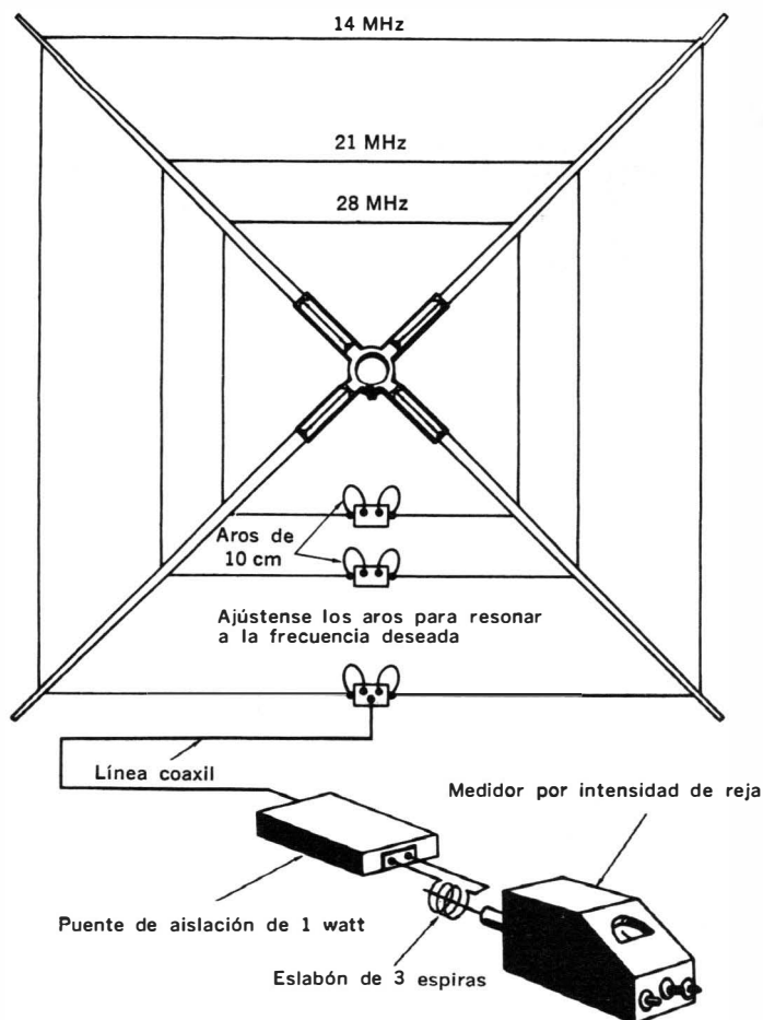
Fig. 7-24. Medición de resonancia desde el extremo de la línea de alimentación.
