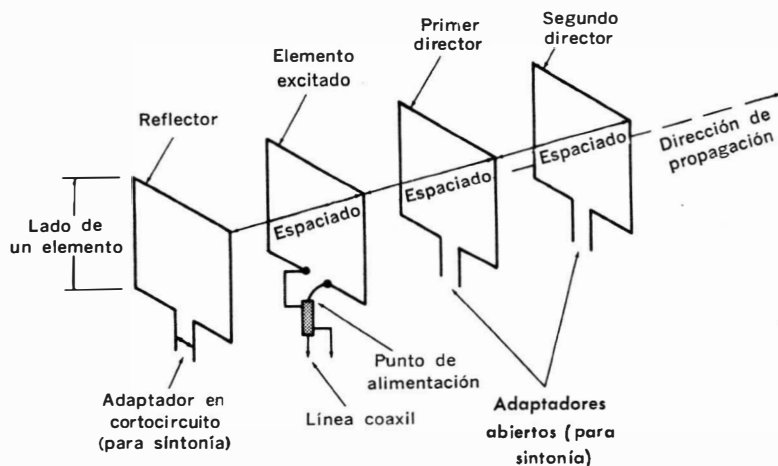
Fig. 7-8. Configuración cuádrice típica de 4 elementos.
