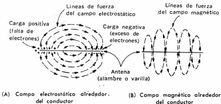
Fig. 2-1. Efectos de capacitancia e inductancia en una antena.
