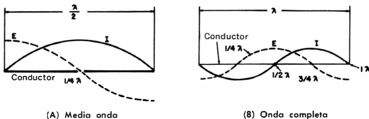
Fig. 3-1. Tensión y corriente de radiofrecuencia en antenas lineales.
