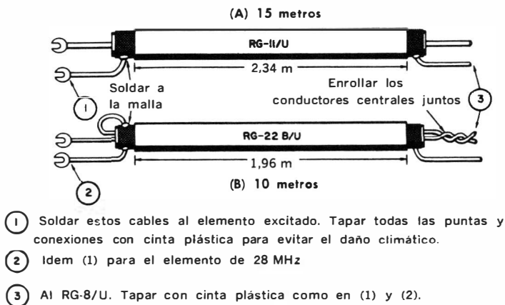
Fig. 7-18. Transformadores coaxiales de adaptación para 21 y 28 MHz.
