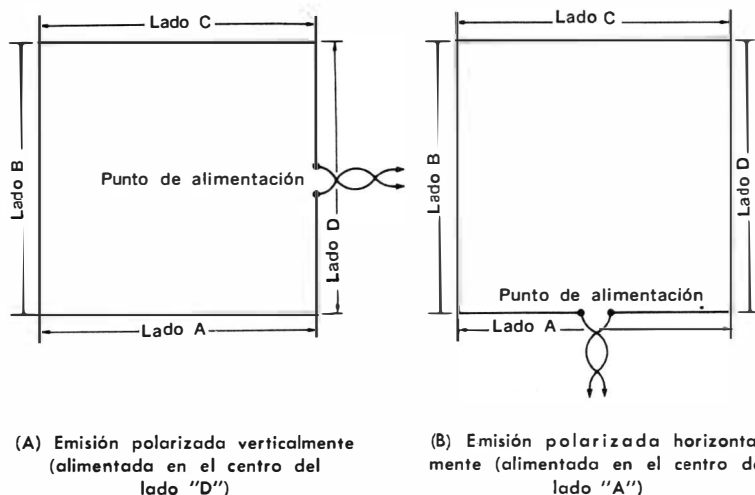
Fig. 7-7. La ubicación del punto de alimentación afecta el comportamiento de la antena cuadrada.
