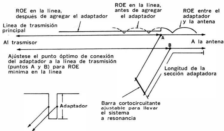
Fig. 5-4. Uso de adaptadores como secciones de ajuste de impedancia.
