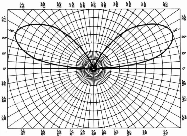
Fig. 3-20. Diagrama de irradiación vertical de una antena longitudinal montado horizontalmente a 0,5 longitudes de onda sobre el terreno
