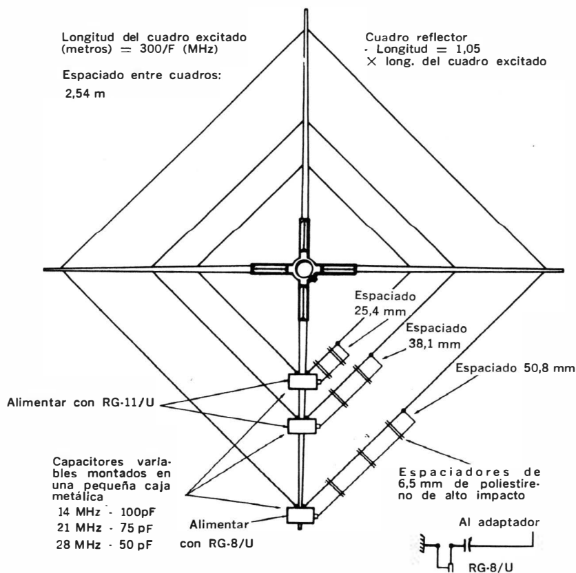
Fig. 7-21. Antena cuadrada de dos elementos, alimentada en "rombo" y con adaptadores gamma para 14, 21 y 28 MHz.
