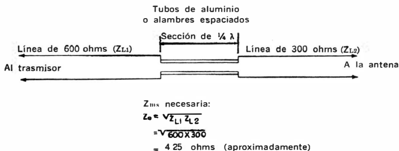
Fig. 5-3. Sección de cuarto de onda utilizada para adaptar líneas desiguales.
