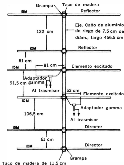
Fig. 7-27. Antena de elementos entrelazados para 10 y 15 metros (para longitudes consultar Tabla 7-1).
