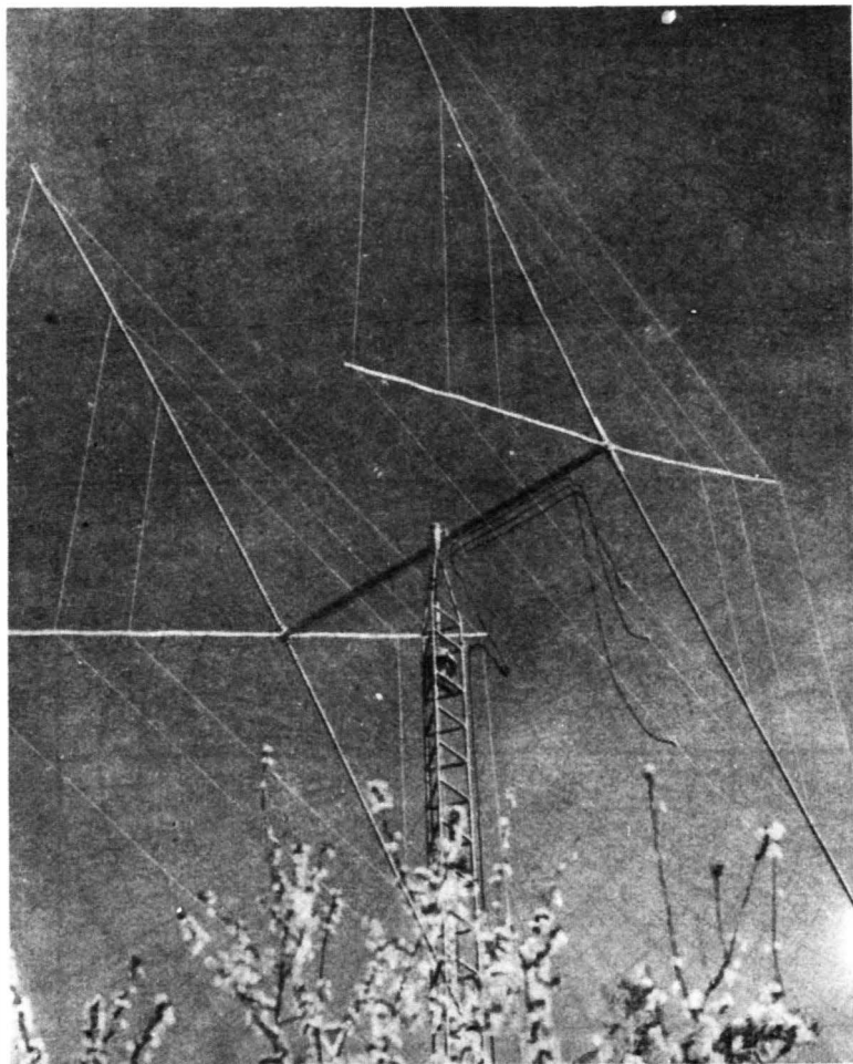
Fig. 3-21. Antena cuádrico cúbico
