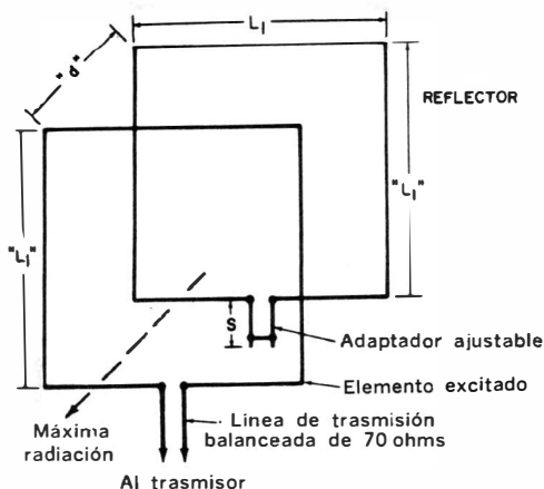
Fig. 3-23. Antena cuádrlica cúbica de dos elementos.
