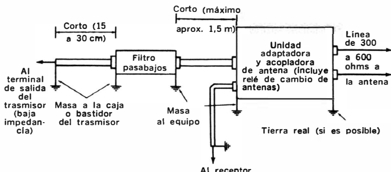
Fig. 6-3. Conexión del filtro pasabajos con el acoplador de antena.
