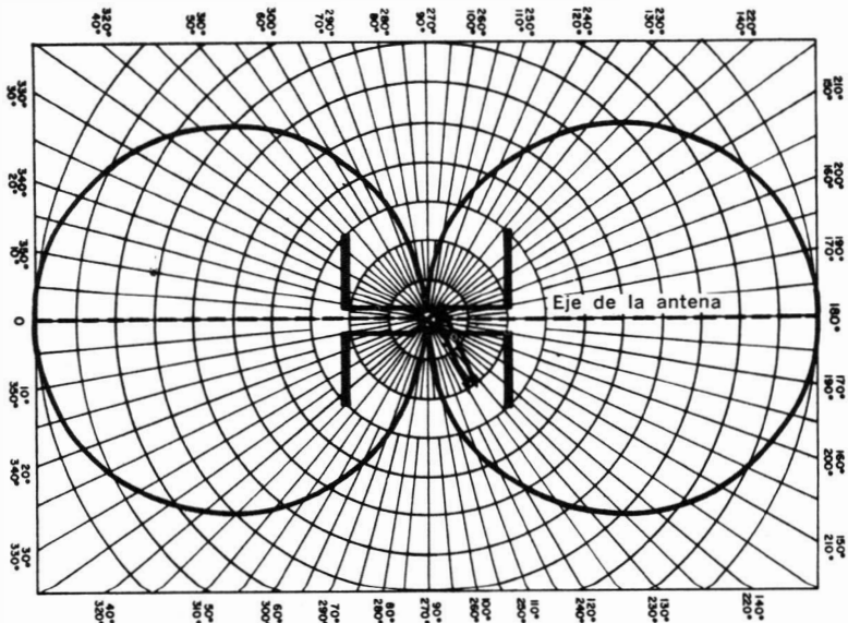
Fig. 3-19. Diagrama de irradiación de una antena activa longitudinal en el plano de los elementos.
