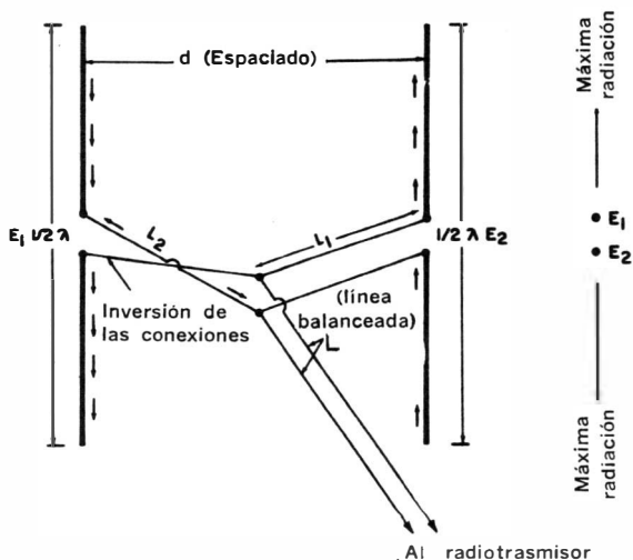
Fig. 3-13. Antena activa con dos elementos de media onda alimentados fuera de fase.
