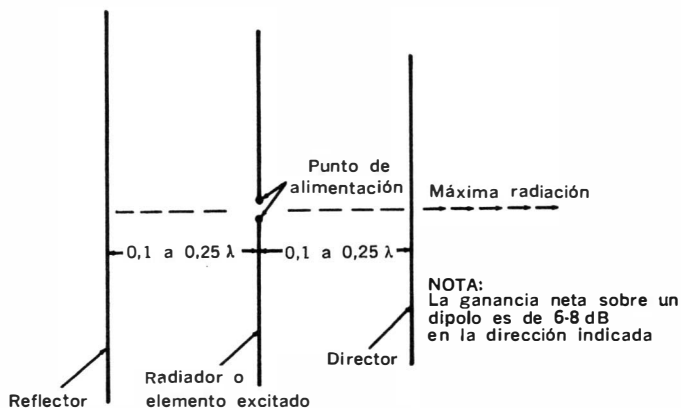
Fig. 3-10. Antena direccional de tres elementos.
