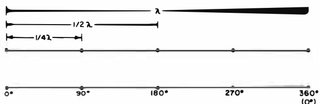
Fig. 4-6. División de una línea de transmisión de onda completa en grados eléctricos.
