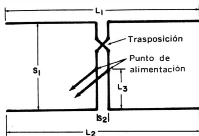
Fig. 3-18. Antena bidireccional longitudinal, activa (8JK).
