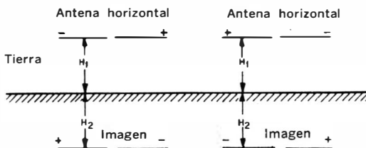
Fig. 2-11. Dipolos de medio ondo y sus imágenes.
