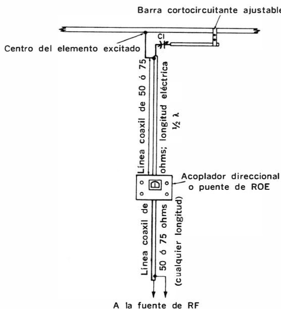
Fig. 5-14. Ajuste del sistema del adaptador gamma.
