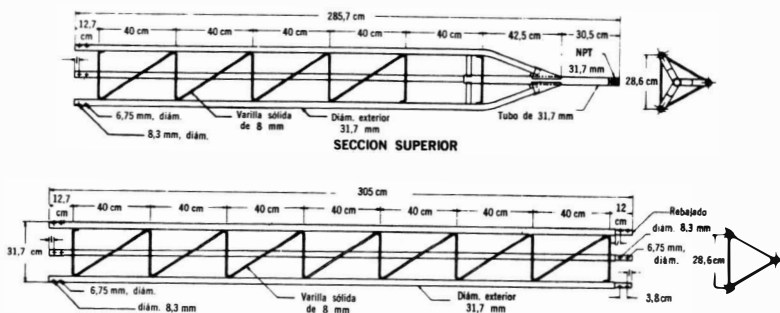
Fig. 8-1. Torre de comunicaciones de uso general.
