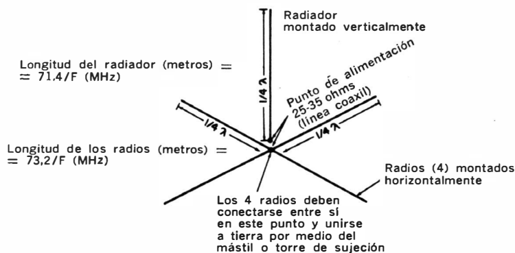
Fig. 3-26. Antena típica con plano de tierra.
