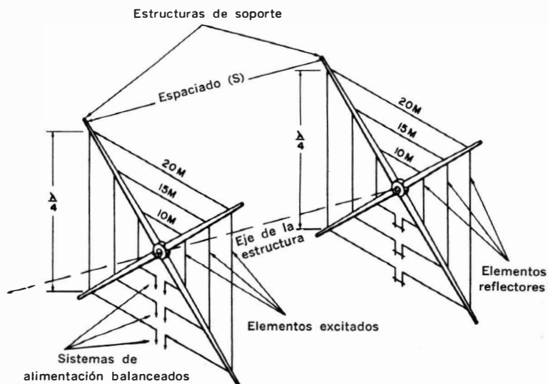
Fig. 7-9. Antena cuádrice multibanda con una sola estructura de soporte.
