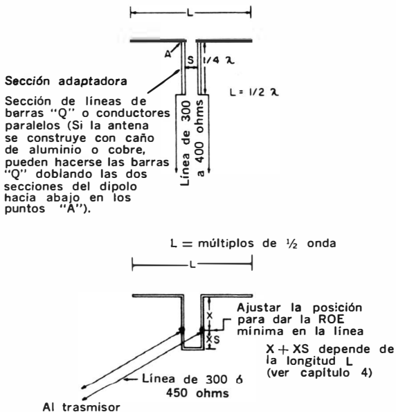
Fig 7-31. Adaptación de una línea de conductores paralelos de 300-400 ohms al elemento excitado.
