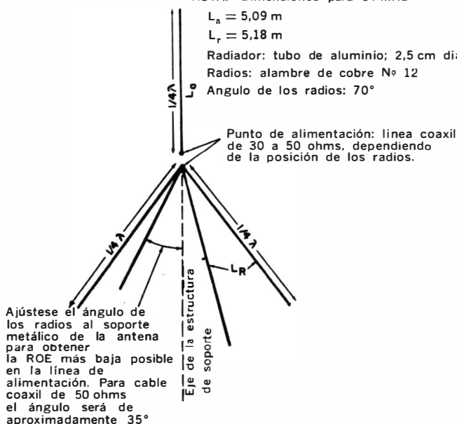
Fig. 3-27. Antena con plano de tierra para FE con radios descendentes
