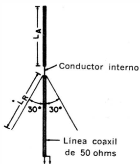
Fig. 3-29. Antena de plano de tierra para las bandas de FME.
