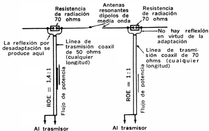
Fig. 4-2. Líneas de transmisión que alimentan dipolos resonantes de media onda (adaptadas y desadaptadas).
