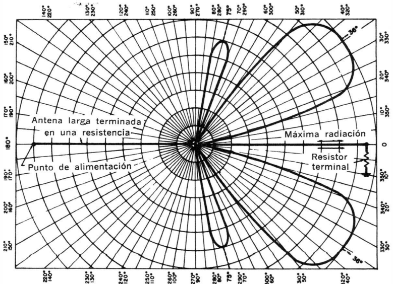
Fig. 3-5. Diagrama de irradiación de una antena larga alimentada en un extremo y terminada en Z_L .
