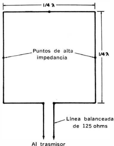
Fig. 3-22. Cuadro básico de las antenas cuádradas.
