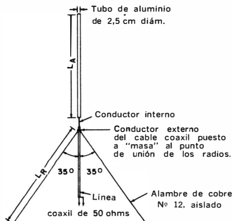
Fig. 3-28. Antena con plano de tierra para bandas de FE.
