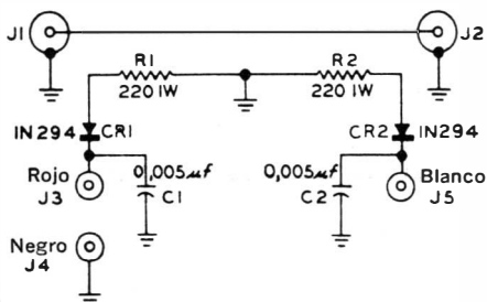
Fig. 6-8. Circuito del acoplador direccional de la Johnson.
