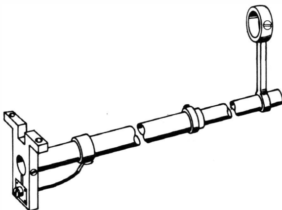
(C) Adaptador gamma de capacitores concéntricos para 6, 10, 15 y 20 metros
