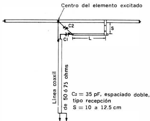
Fig. 5-16. El adaptador gamma modificado.
