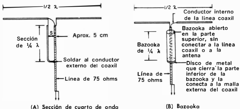
Fig. 7-32. Dispositivos balanceadores para antenas de FME (VHF).
