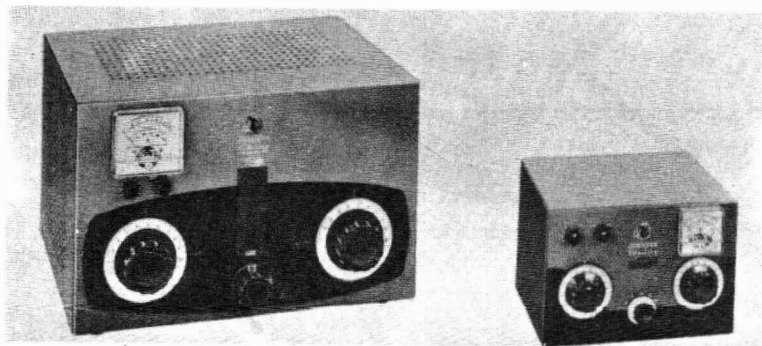
Fig. 6-6. Dispositivos de acoplamiento y ajuste de antena, totalmente integrados
