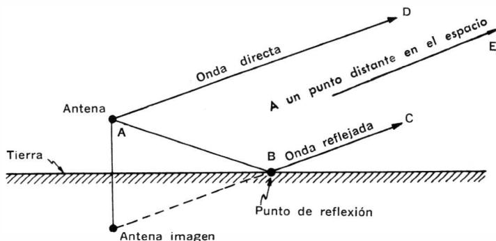
Fig. 2-9. Ondas directa y reflejada provenientes de una misma antena.
