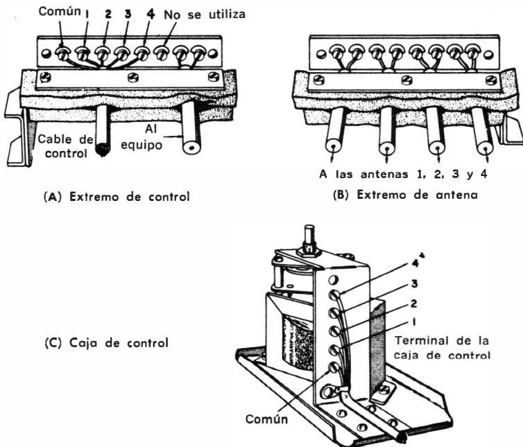
Fig. 7-17. Conexiones de la llave remota de antena TS-4.
