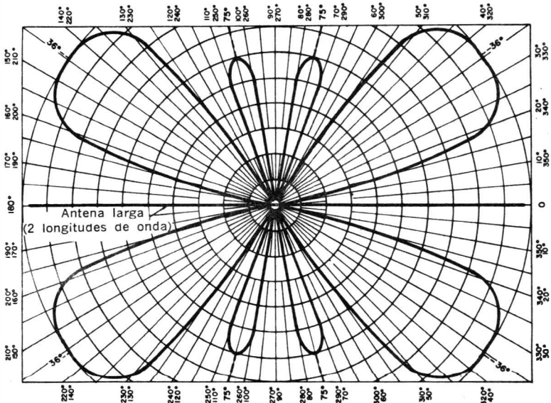
Fig. 3-4. Diagrama de irradiación de una antena de dos ondas completas.
