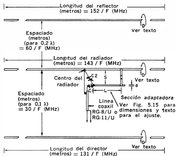
Fig. 7-2. Antena parasitaria sencilla de tres elementos.
