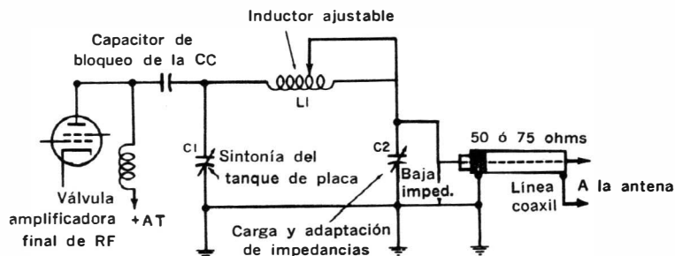
Fig. 6-1. Acoplador en pi para el circuito de salida de los transmisores modernos.
