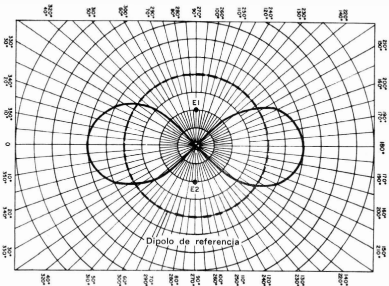
Fig 3-12. Diagrama de irradiación de dos elementos de media onda alimentados en fase.
