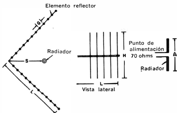
Fig. 3-35. Diagramas básicos de antenas tipo reflector esquinero.
