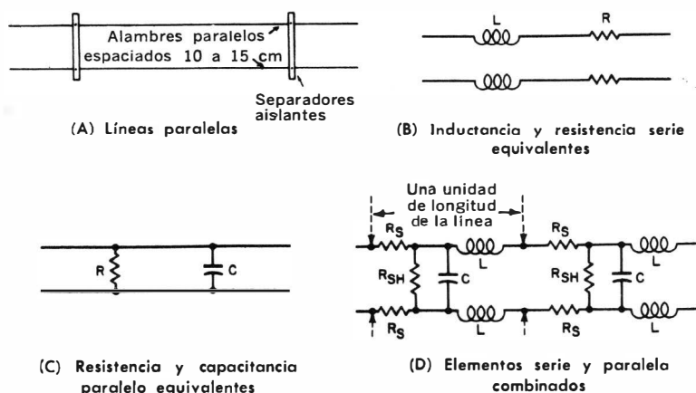
Fig. 4-4. Constantes RLC distribuidas en una línea de transmisión.
