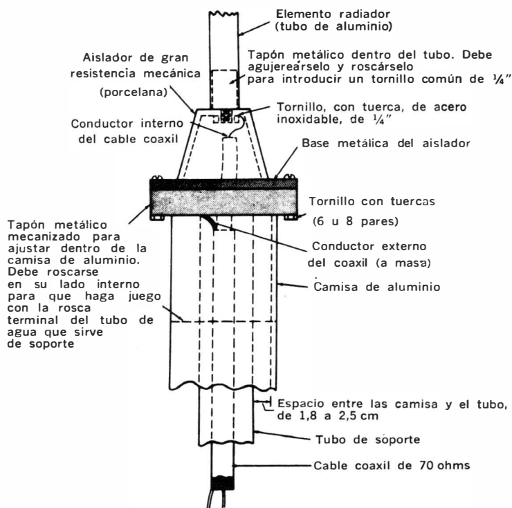
Fig. 3-31. Detalles de la estructura del punto de alimentación.
