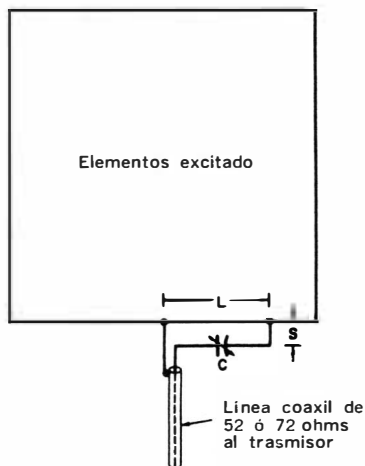
Fig. 7-22. Dimensiones y valores de los capacitores para las secciones gamma de la Fig. 7-21.
