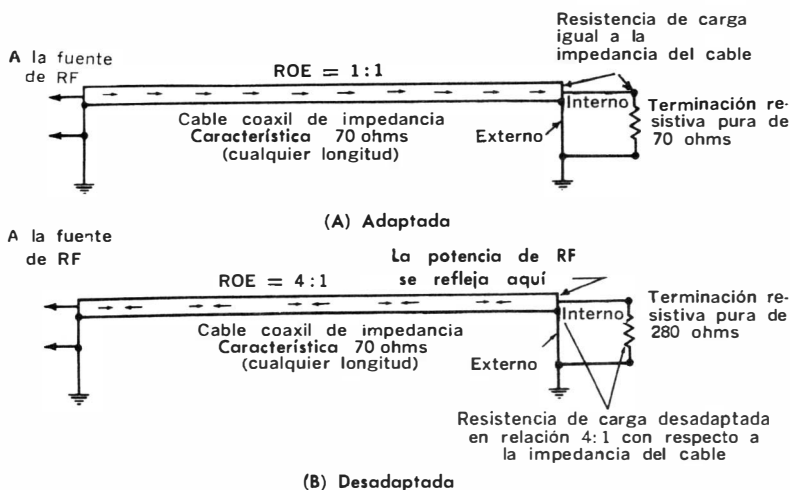
Fig. 4-1. Reflexión de RF (y alta ROE) en una línea de transmisión.
