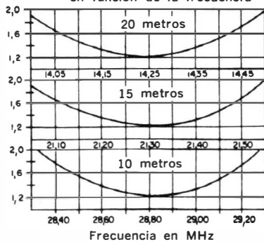
Fig. 7-6. Antena Telrex para servicio pesado.
