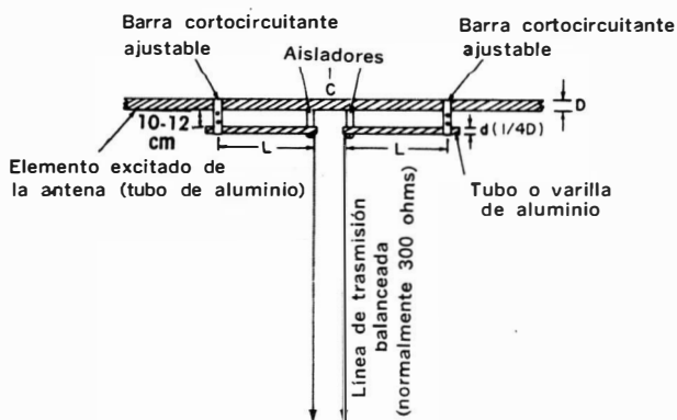
Fig. 5-11. Adaptador T.
