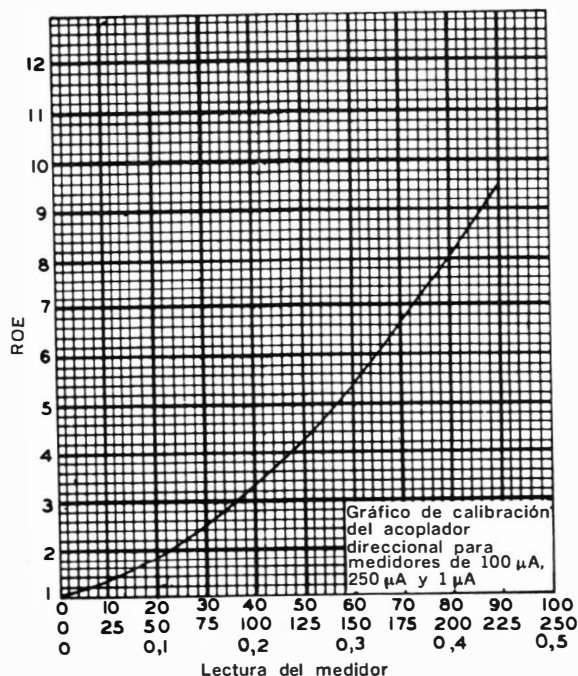
Fig. 6-10. Carta de calibración del acoplador direccional para instrumentos de 100 y 250 microamperes, y 1 miliampere.
