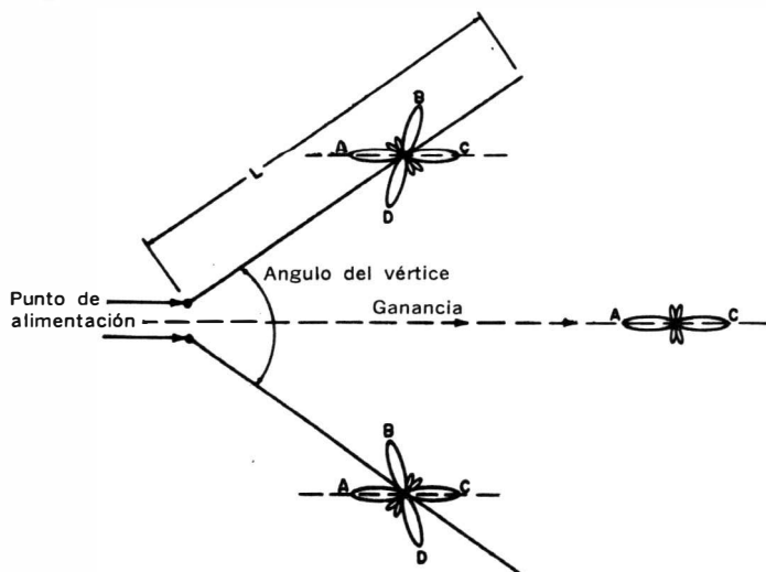
Fig. 3-6. Antena en V.
