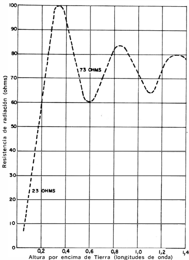
Fig. 2-13. Resistencia de irradiación de una antena dipolo de media onda alimentada al centro.
