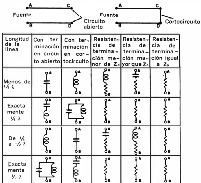
Fig. 4-9. Circuitos equivalentes de una línea de transmisión con distintas terminaciones.
