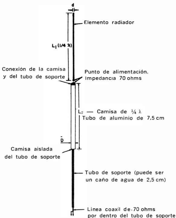
Fig. 3-30. Antena vertical de media onda tipo "camisa"
