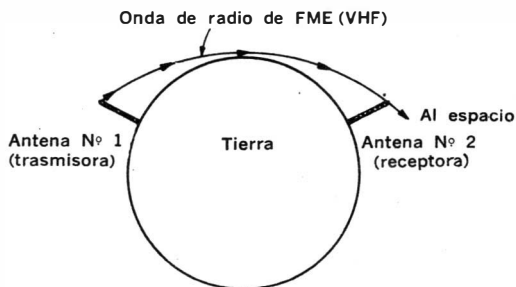
Fig. 1-5. Extensión de la distancia al horizonte y de la distancia de alcance visual por la curvatura de las ondas.
