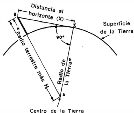
Fig. 1-4. Cálculo geométrico de la distancia al horizonte de una antena.
