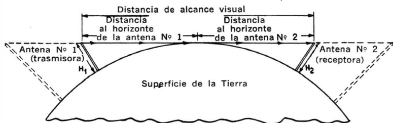
Fig. 1-3. Distancia de alcance visual y distancia al horizonte.
