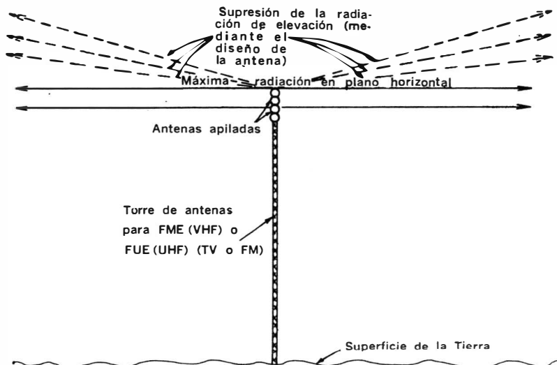
Fig. 1-2. Propagación por línea directa desde una antena de TV o FM.
