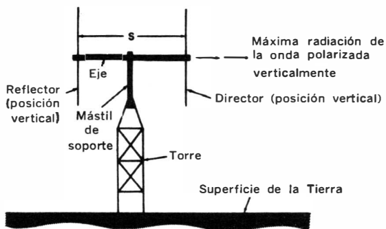
Fig. 3-25. Antena parasitaria montada verticalmente.
